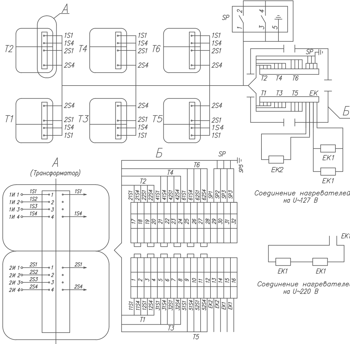
Рисунок 4. Схема вторичных цепей выключателя ВГБ-35, I ном =1000 А
